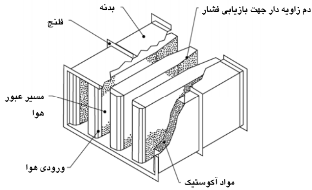
صدا خفه کن (Sound Attenuator)
