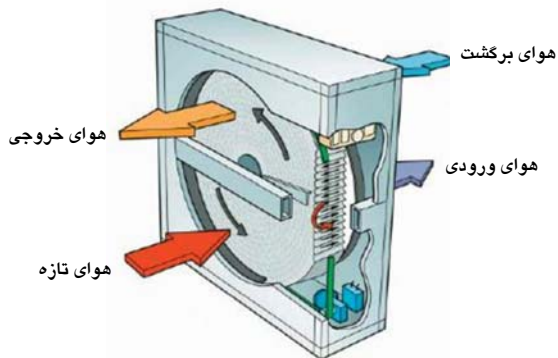
چرخ بازیافت حرارت (Heat Recovery Wheel)
