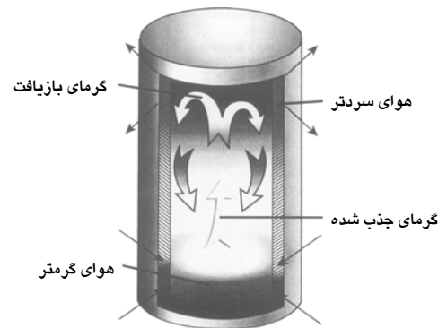
لوله حرارتی (Heat Pipe)
