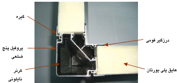
سپر حرارتی (Thermal Break)
